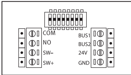
Detailansicht Anschlusspanel
